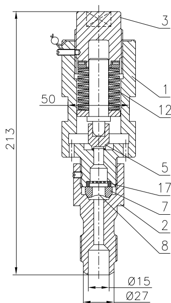
Rys. 1 Bezpiecznik ciśnieniowy
