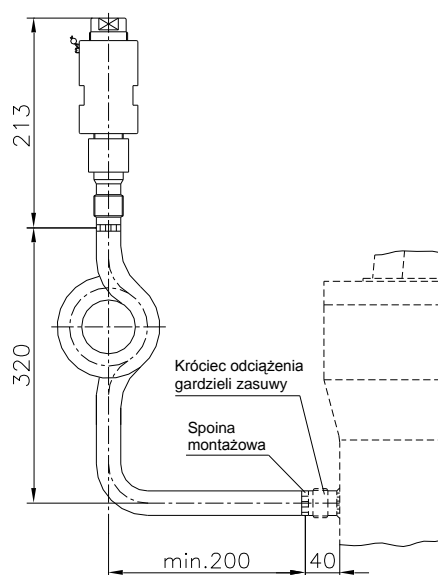
Rys. 2 Zespół bezpiecznika ciśnieniowego
